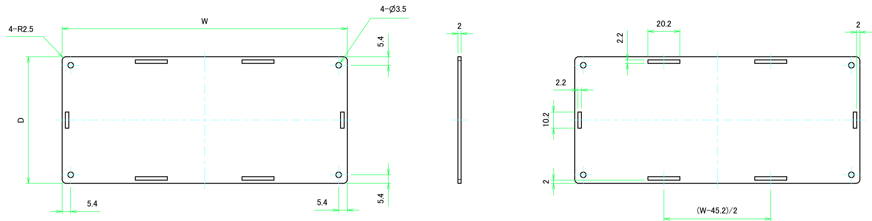
上カバー裏面 / Top cover Backside
