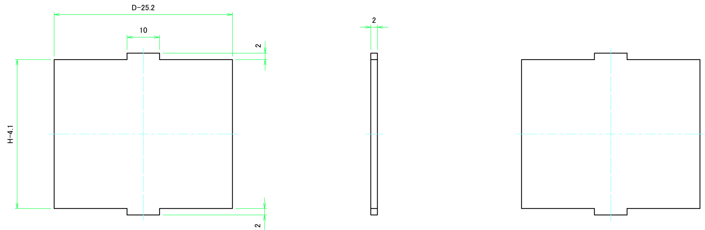
Dパネル1表面 / D Panel 1 Frontside
